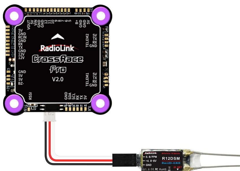
乐迪 R12DSM 接收机连 CrossRace Pro
