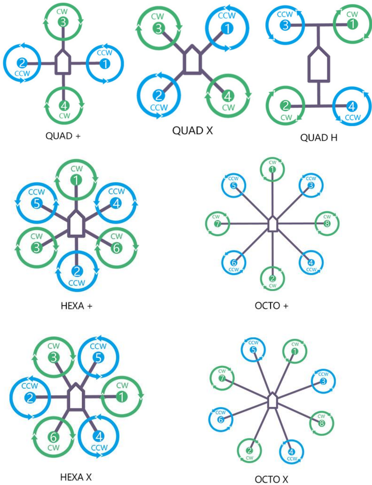
机架安装电机转动方向图：
