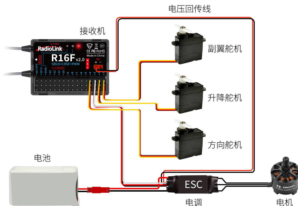
R16F 接收机电压回传连接示意图
